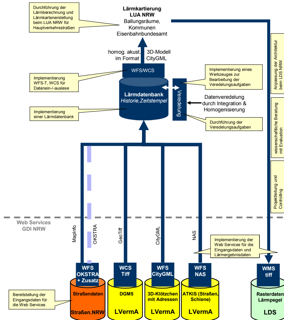
Abb. 2: Hauptaufgabenpakete zur technischen Umsetzung der Umgebungslärmkartierung in NRW (Graphik: IKG Uni Bonn).
