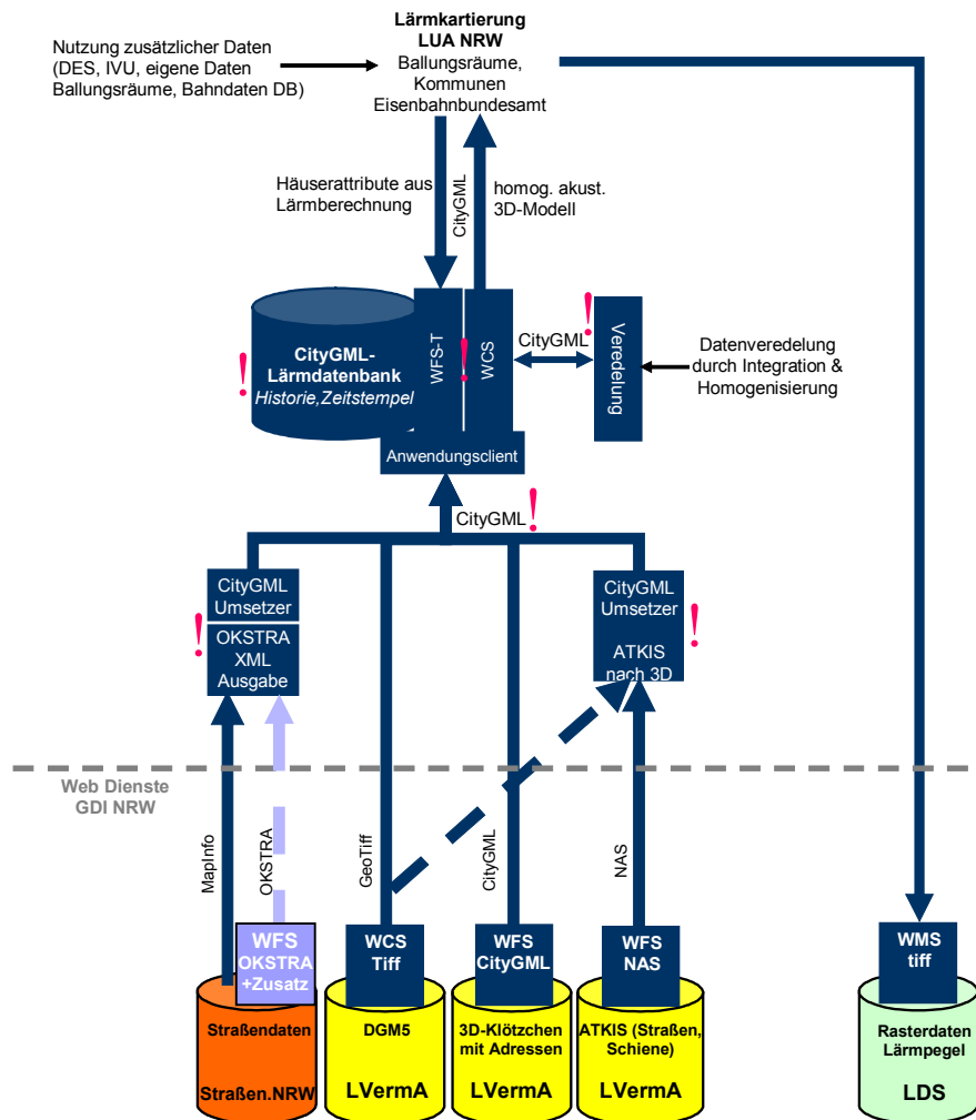
Abb. 3: Empfohlene Systemarchitektur (Graphik: IKG Uni Bonn).
