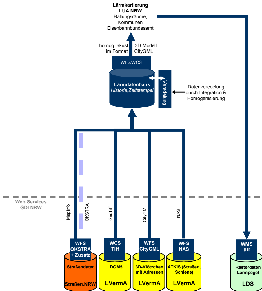
Abb. 1: Grundarchitektur der technischen Umsetzung der Umgebungslärmkartierung in NRW mit den wichtigsten Komponenten (Graphik: IKG Uni Bonn).
